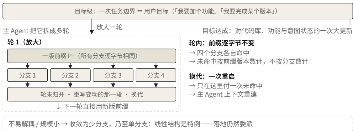
图3 两个尺度。目标级由用户给出（一次任务边界），主Agent把它拆成多轮；轮级由归并触发——一轮结束、前缀换代，主Agent的上下文随之重建。一轮之内前缀不换版本，所以那一版只在换代时付一次未命中。不易解耦或规模小的时候，分支数可以收敛到一：那是线性结构，而线性是这个循环结构的特例——落地仍然委派。数据源：正文“具体实现”一节。
